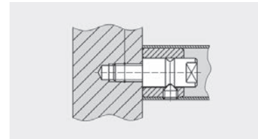
MIM-432-00-121 GZ 234 Çerçevesi kapılar için (20mm vida derinliği) Tek tarafli bağlantı elemanı
