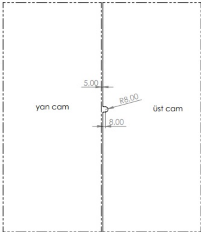
CAM KESİDİ
